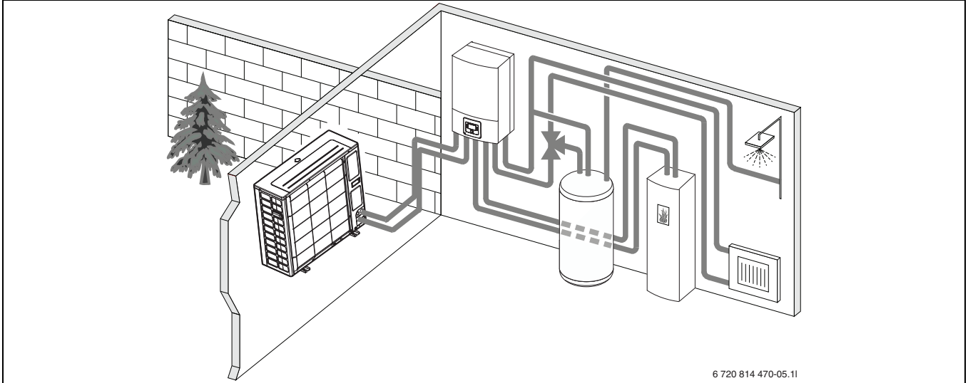
Kuva 3 Lämpöpumppu ulkoyksikkö, sisäyksikkö AWBS ilman sähkölisälämmittintä ja ulkoista lämminvesivaraajaa
