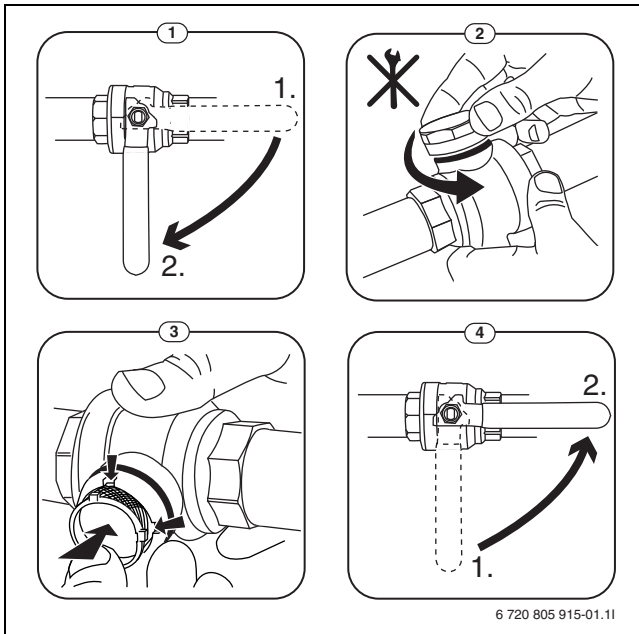
Kuva 5 Suodatinvaihto ilman lukkorengasta
