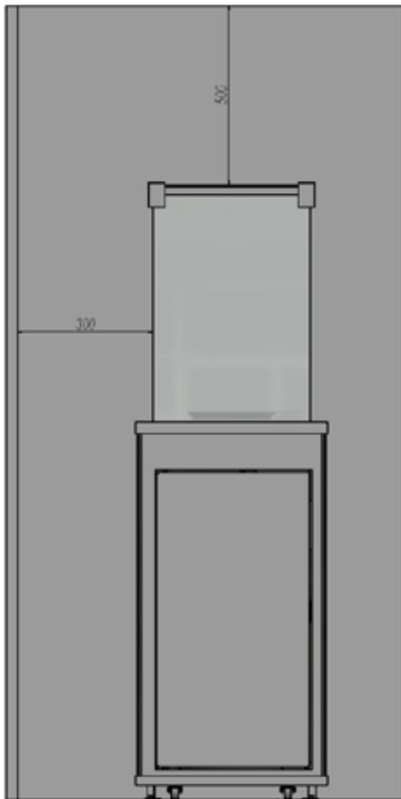
Рис.6. Минимально допустимое расстояние до легковоспламеняющихся материалов
