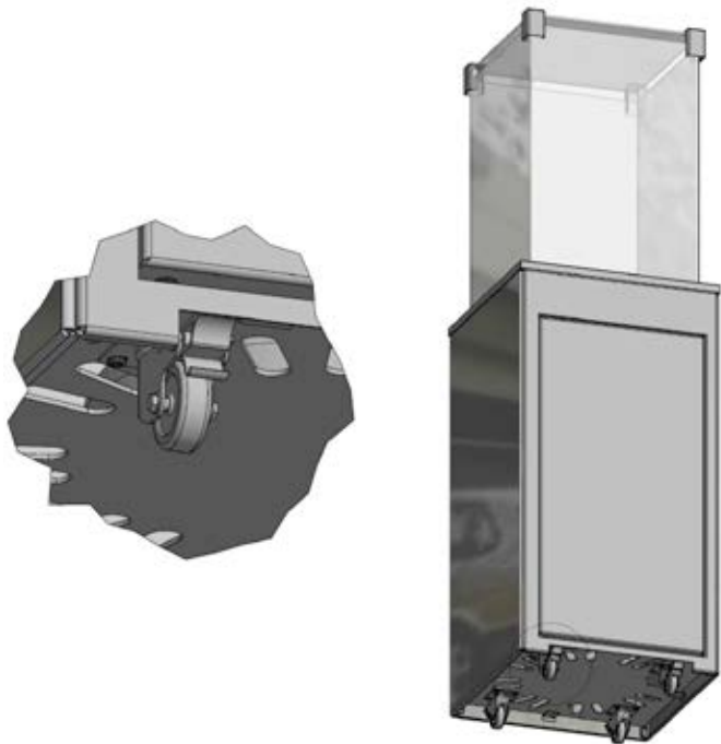
Рис.2. Колеса с блокираторами для облегчения движения и надежной фиксации в стационарном положении.
