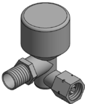
Abb. 8. Das in der Anlage installierte Anti-Kipp-Sicherheitsventil.
