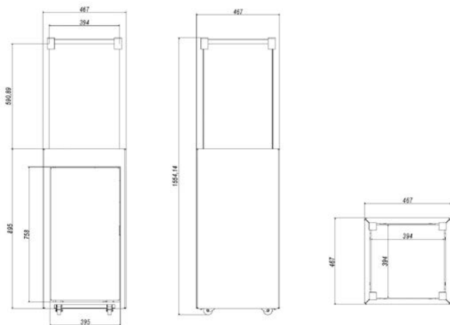
Рис.1. Схема нагревателя PATIO с размерами
