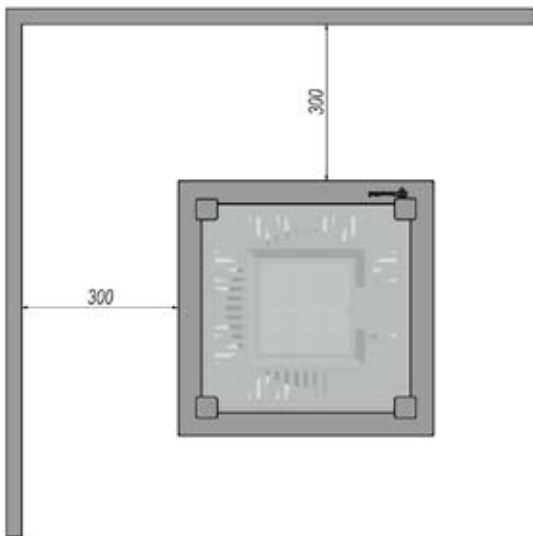
Abb. 3 Minimaler freier Bereich von leichtentzündlichen Stoffen/Gegenständen
